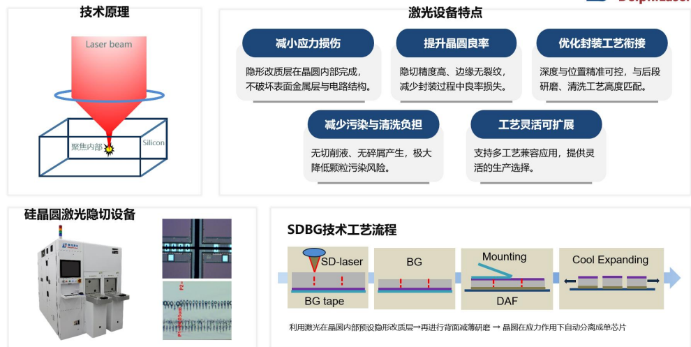
图 4 公司硅晶圆激光隐切设备与 SDBG 技术工艺流程
